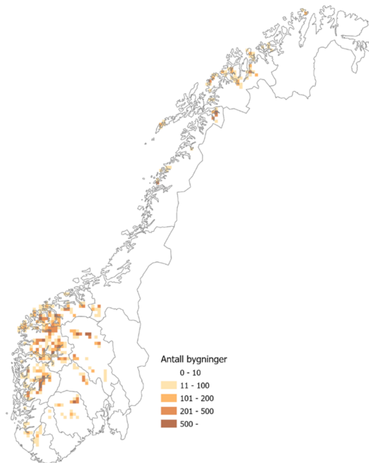
Figur 2 Antall bygninger i områder med fare for 1000-års- og 5000-årsskred i bratt terreng i 2019 (en rute er 10 x 10 km); fylkesgrensene er grensene til og med 2019
